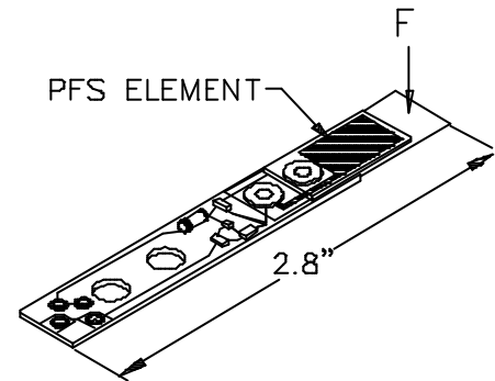
Smart Switch SW100
